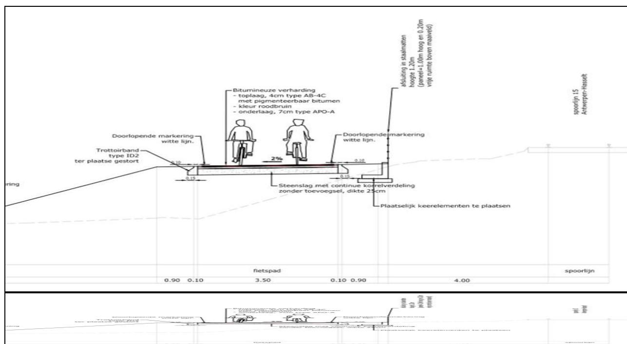
Figuur 4: type dwarsprofiel fietsostrade
