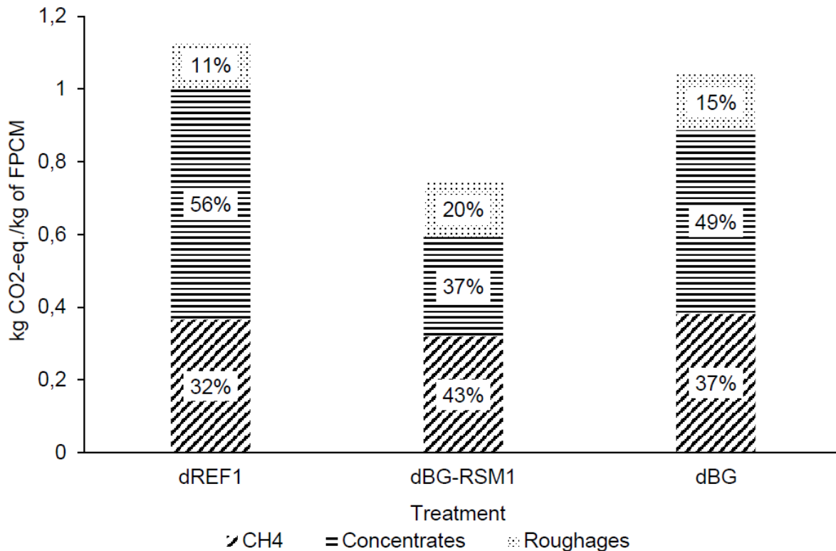
Figuur 8: Koolstofvoetafdruk bij een controle rantsoen dREF1 (MKV, VDK, PP, sojaschroot en krachtvoeder) tov van eenzelfde rantsoen met bierdrاف and koolzaadschroot (dBG-RSM1) en een rantsoen met enkel bierdrاف (dBG) (bron: ILVO).
